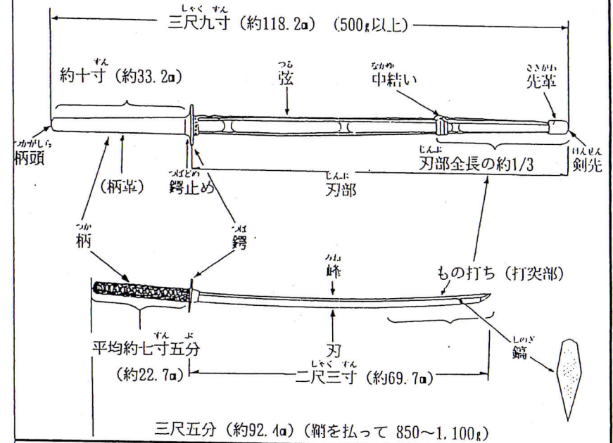
竹刀の各部位の名称と刀との比較 (成人男子用)
